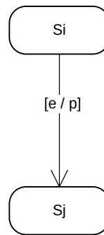
6. ábra: EDFSM-beli állapotátmenet
