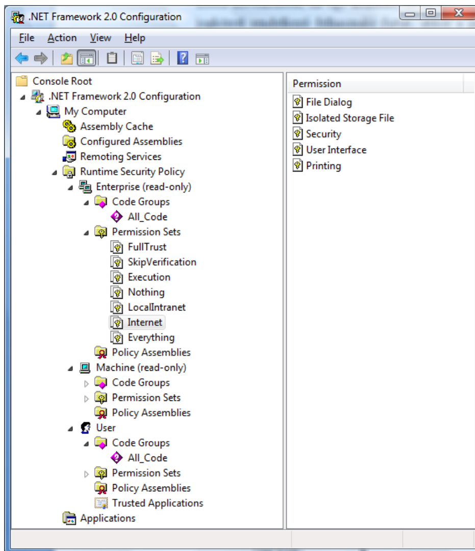
1. ábra: A .NET futás idejű biztonsági házirendje
