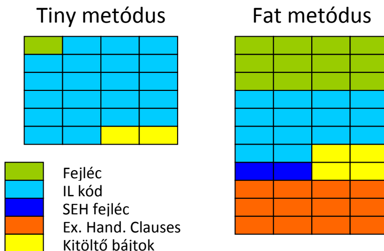
29. ábra: .NET metódusfajták kategorizálása
