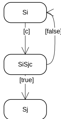
7. ábra: DFSM-ben értelmezett állapotátmenet
